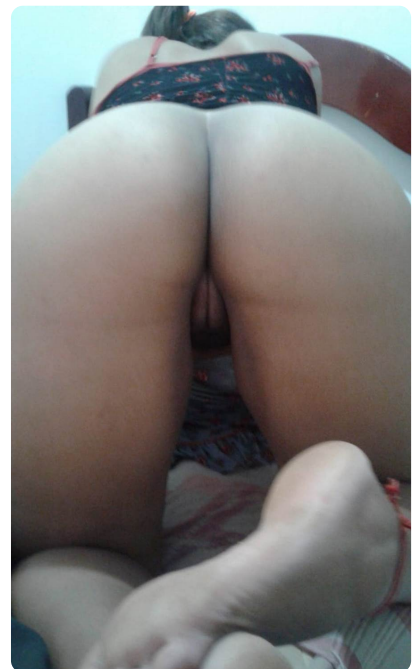
ComfyUI.
